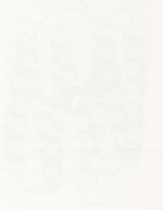
Figuur 1. Structuur van het membraan eiwit beta-galactosidase, met daarboven het cytoplasma en de extracel- lulaire ruimte. De structuur is gebouwd met 2 dimensie-eiwitten met behulp van een membraan. Ze zijn op 3- dimensie- eiwitten die door moleculaire modellen met elkaar verbonden zijn.
