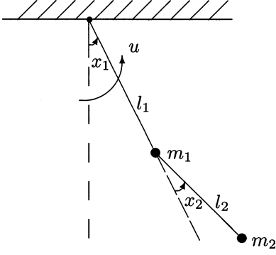
Fig. 1. Double pendulum.
