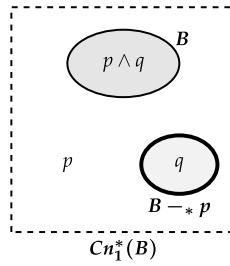
Fig. 1. Cn_1^* in Example 23.
