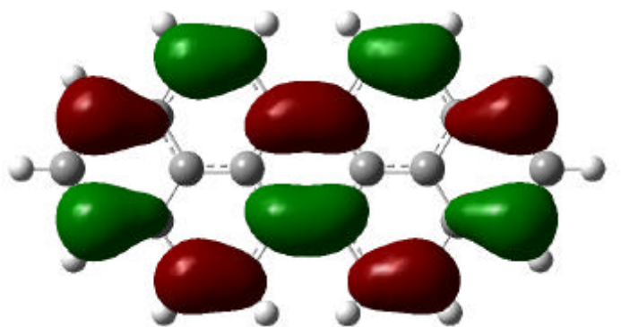
HOMO
