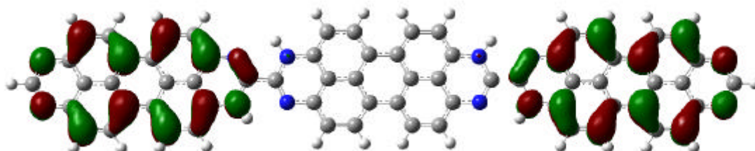
LUMO
